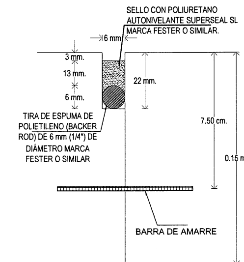
DETALLE 4 DE JUNTA DE CONSTRUCCION LONGITUDINAL (BARRAS DE AMARRE)
