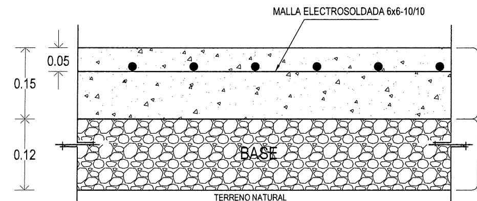
ESTRUCTURA DE PAVIMENTO SIN ESCALA
