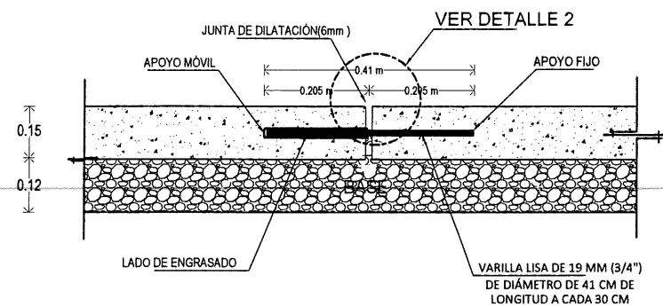
DETALLE DE PASAJUNTAS EN PAVIMENTO RIGIDO SIN ESCALA
