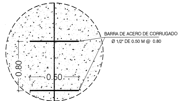
DIMENSIONES EN JUNTAS LONG. CON BARRAS DE ACERO CORRUGADO SIN ESCALA
