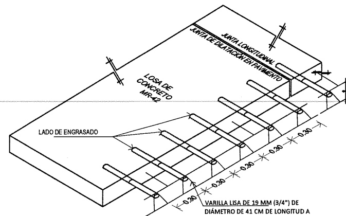
DETALLE ISOMETRICO DE PASAJUNTAS SIN ESCALA
