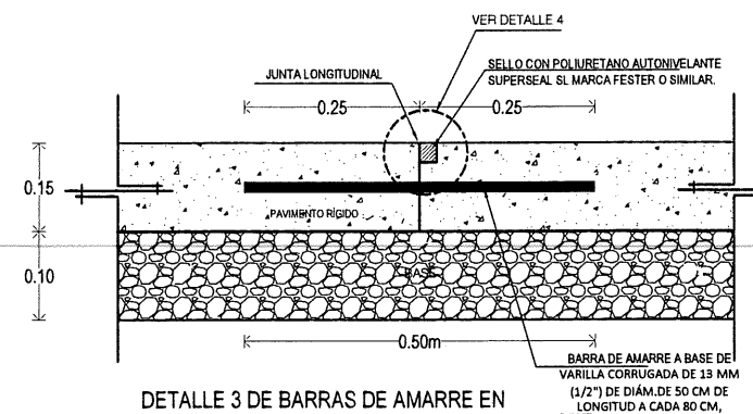
DETALLE 3 DE BARRAS DE AMARRE EN PAVIMENTO RIGIDO
