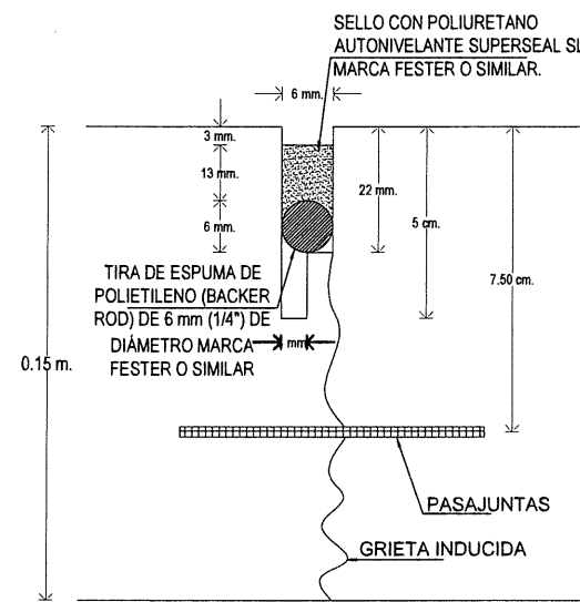
DETALLE 2 DE JUNTA TRANSVERSAL SIN ESCALA
