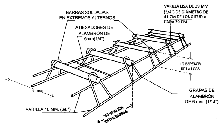
ISOMETRICO DE CANASTILLA PASAJUNTA SIN ESCALA
